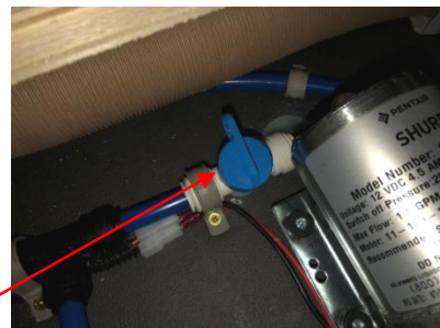
Vanne de vidange d'eau propre
