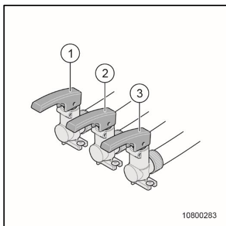
Fig. 158 Robinets de vidange de diminution du poids, du chauffe-eau et d'eau fraîche
