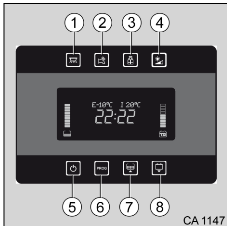
Fig. 118 Panneau de contrôle
