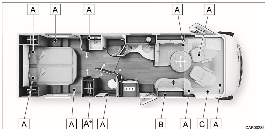
Fig. 180 Emplacements sur la variante avec lit central et salle de bain XL
