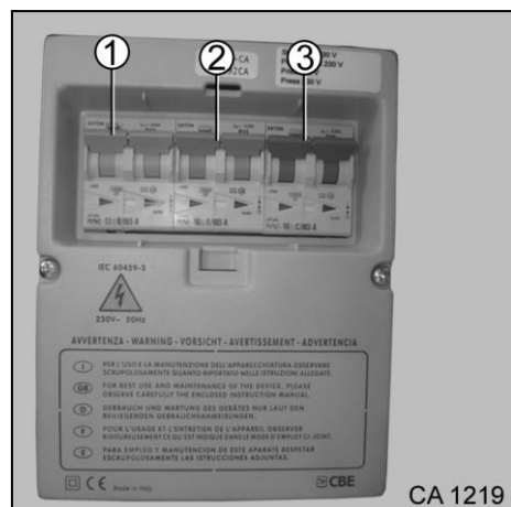
Fig. 114 Disjoncteur FI
