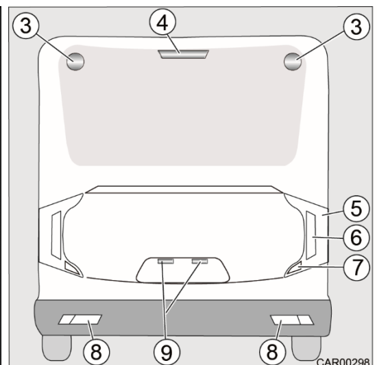
Fig. 195 Éclairage arrière
