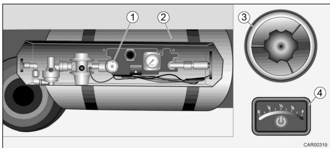
Fig. 129 Réservoir de gaz, bouchon de carburant et téléaffichage
